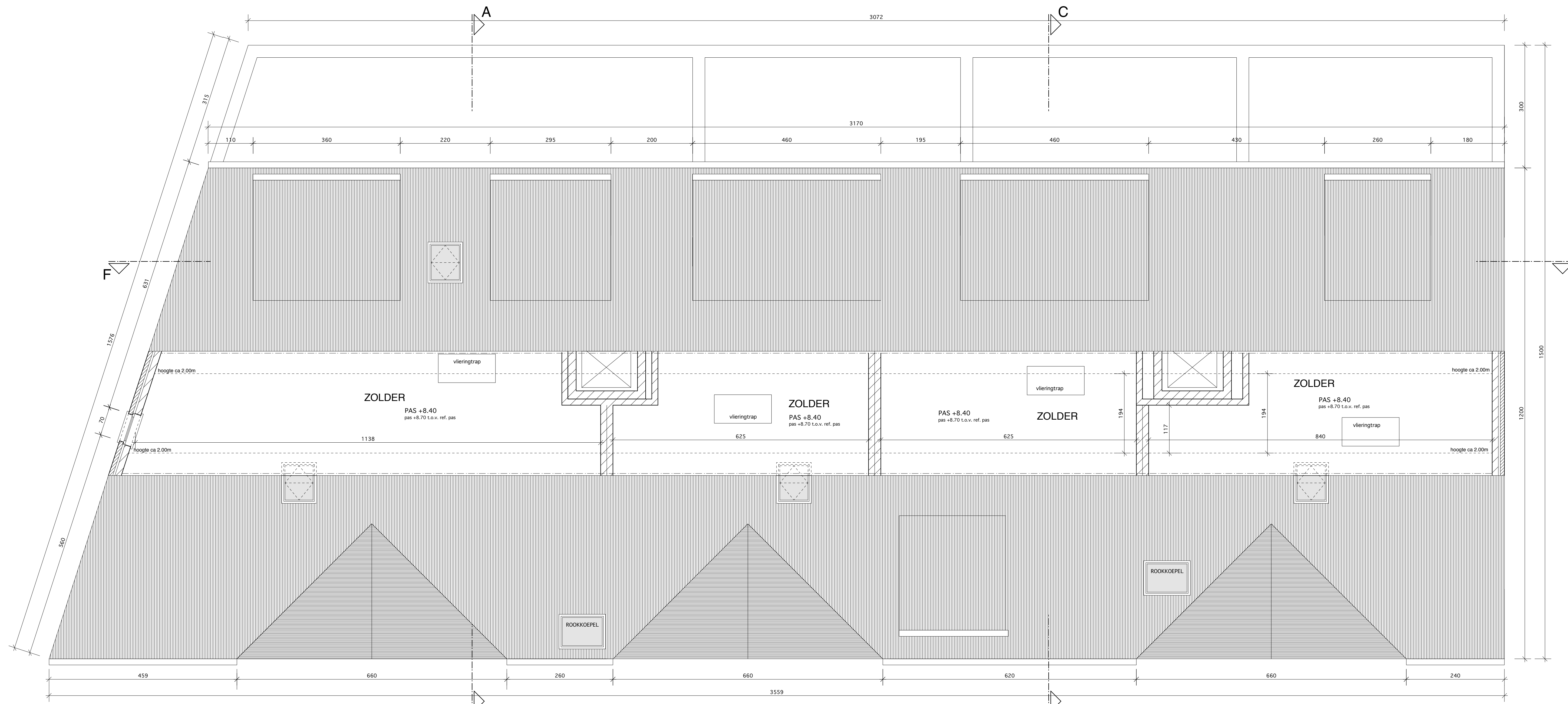
PLANZICHT ZOLDERVERDIEPING
